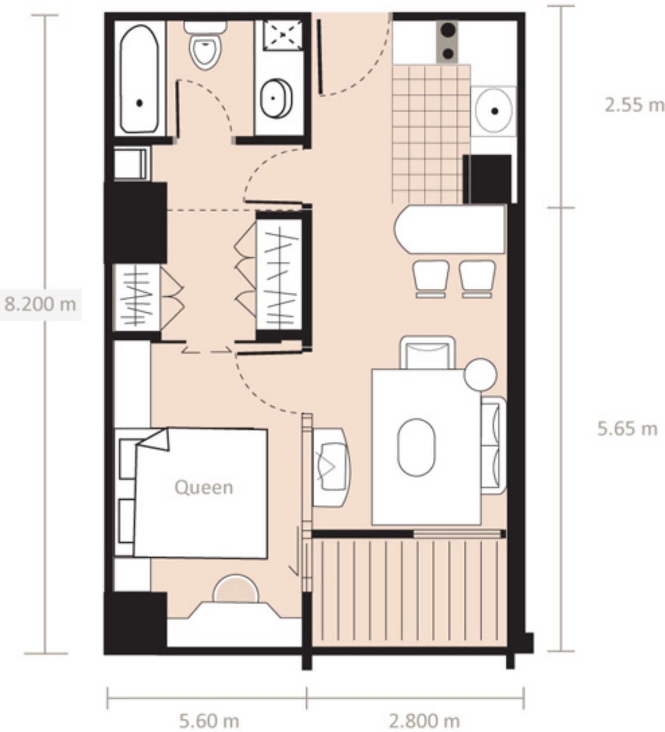
Floor plan Junior Suite (B)
